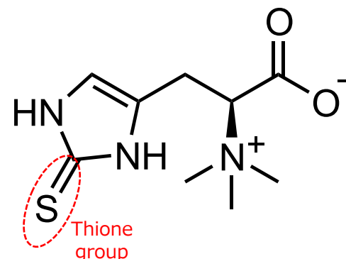
Fig. 1. L-Ergothioneine (EGT)
